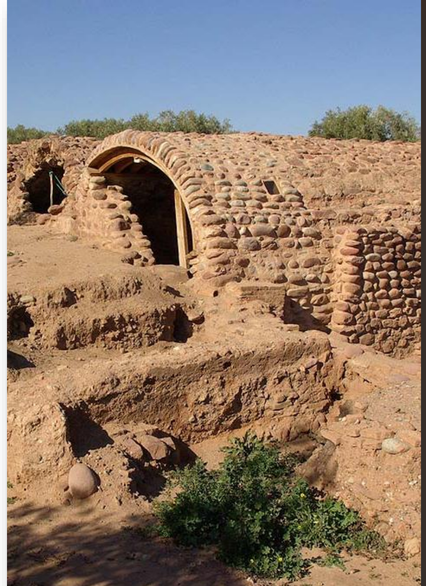
La structure voûtée du hammam Photo I. Six – https://darzampa.wordpress.com/2012/06/02/112/
